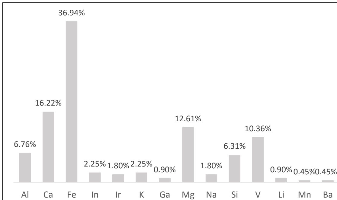
Figura 1. Resultados de análisis de muestras de rocas valle de Chao.
