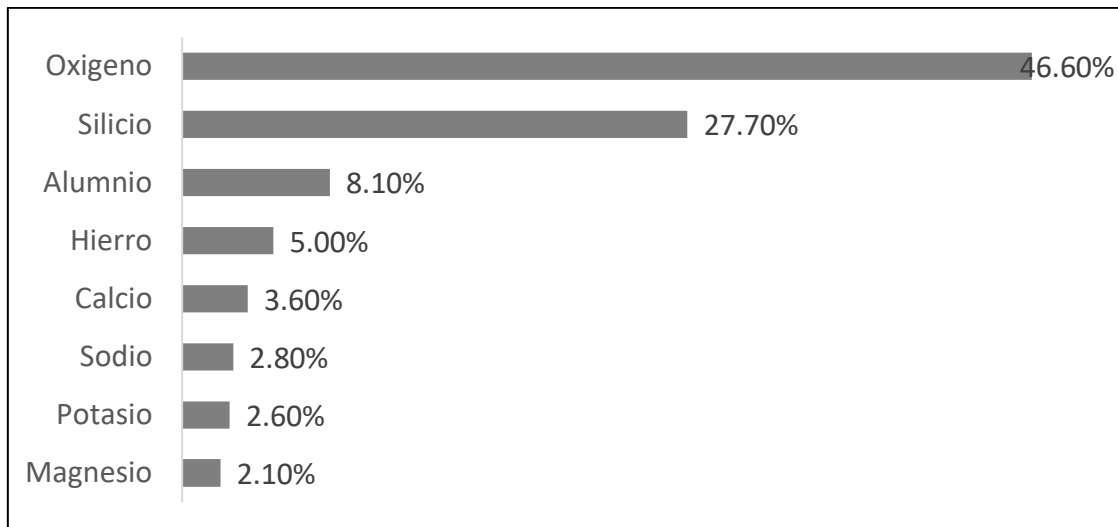
Figura 5. Elementos abundantes en la corteza terrestre Tarback y Lutgens (2005)
