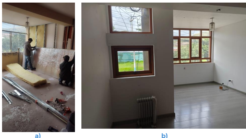
Figura 12. Implementación de la envolvente térmica en piso, muros interiores y techo. a) Muros interiores con trasdosado de sistema drywall conformado por EPS, lana de vidrio, barrera de vapor y placa de yeso. b) Piso con espuma aislante y piso laminado HDF (8.3 mm, 19.3x1.20 cm); cambio de ventana a sistema de aluminio con vidrio doble (6 mm) con cámara de aire sin rotura de puente térmico; techo con cielo raso de EPS (1"). Fuente: elaboración propia.
