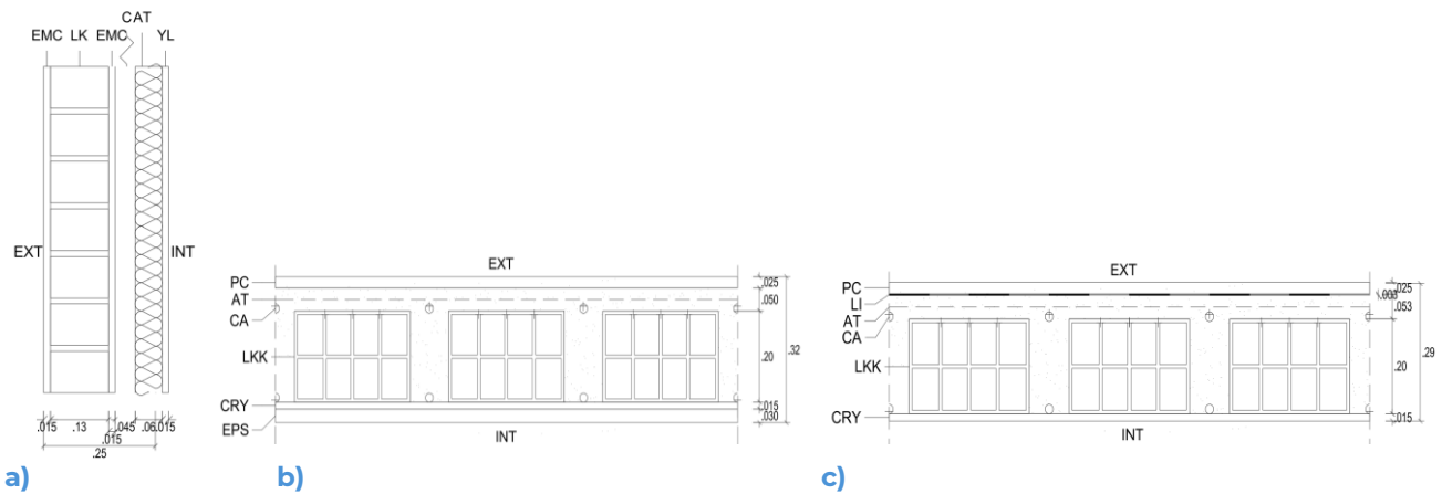
Figura 10. Detalle constructivo envoltente térmica. a) Muro trasdosado interior donde: INT=interior, YL= placa de yeso, AT= aislamiento térmico lana de vidrio con para vapor, C=cámara de aire, EMC=enlucido mortero cemento, EXT= exterior. b) Techo donde: EXT= exterior, PC=piso flotante, AT= Aislamiento térmico, CA= Concreto armado, LKK= Ladrillo King Kong para techo, CRY=cielo raso de yeso, EPS=Poliestireno expandido. c) Piso donde: EXT= exterior, PC=piso flotante, Li= espuma de poliestireno, AT= Aislamiento térmico, CA= Concreto armado, LKK= Ladrillo King Kong para techo, CRY=cielo raso de yeso. Fuente: elaboración propia.
